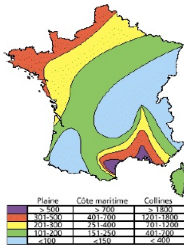
Puissance moyenne du vent en W pour un m2 de section verticale prise à 50 m du sol. Source ADEME
