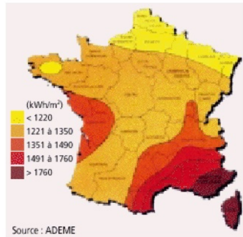
Energie solaire reçue par m2 et par an en France. Source ADEME.
